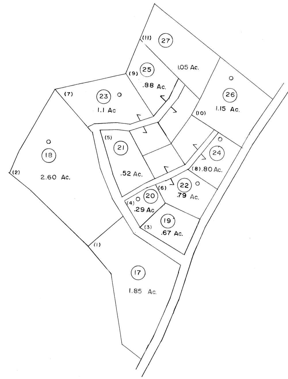
INSET A SCALE: 1" = 200'
