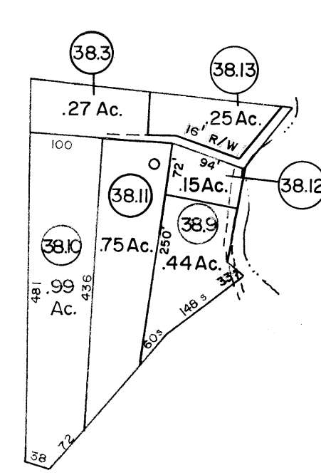
INSET #1 SCALE: 1" = 200'
