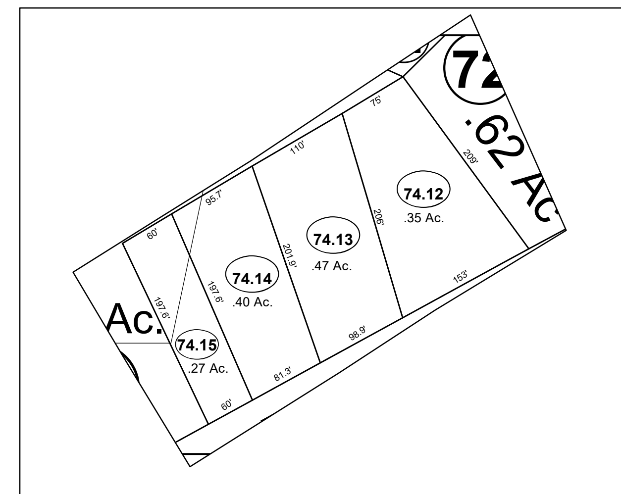
Insert "C" Scale: 1 inch equals 100 feet
